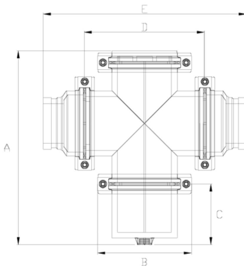
ITEM 521 | Filtro cazapiedras s/Netvitc®
